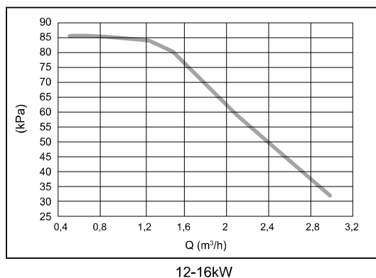
Presión estática externa disponible VS Caudal
